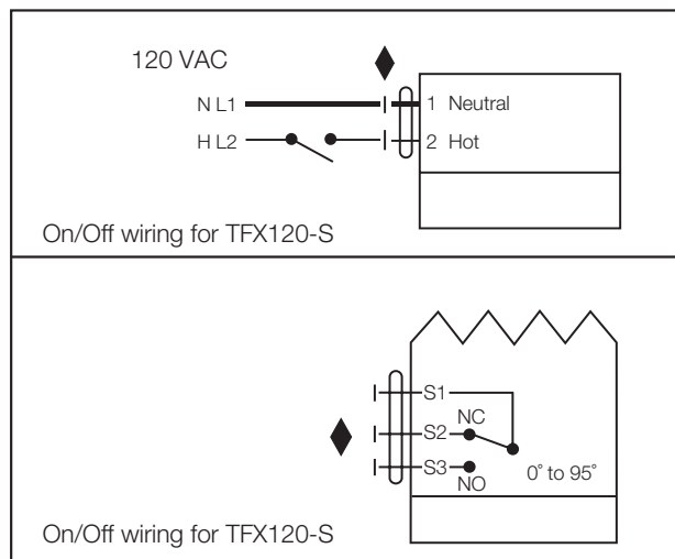
Fig. 4 120 VAC Actuator
