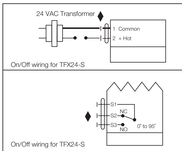
Fig. 5 24 VAC/VDC Actuator
